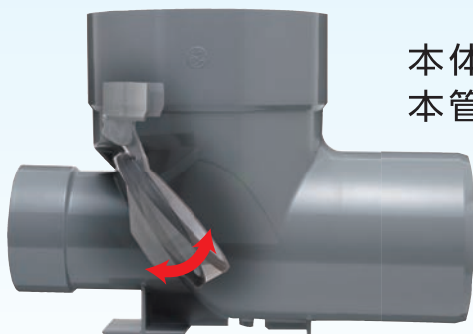
逆止弁付公共マス KG-S150P×100-200
